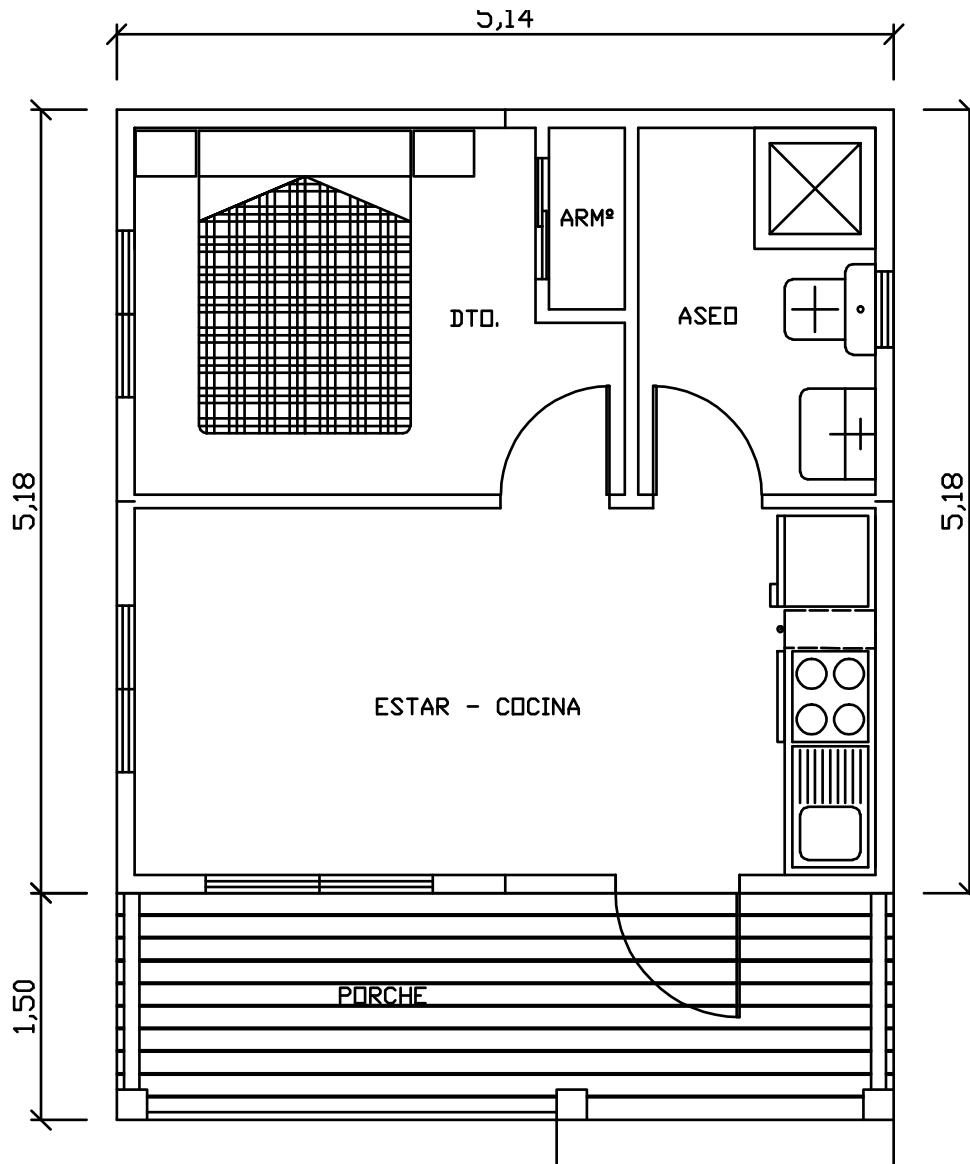
PLANTA
